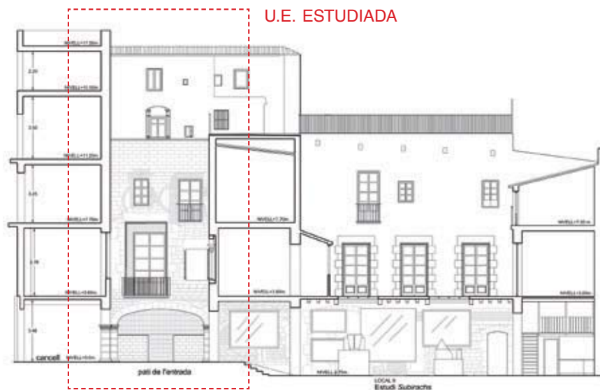
Figura 38. Aixecament estat actual. C/ del Regomir, núm. 11-19. Secció AA'. Vegeu la línia de secció a la figura 30.
