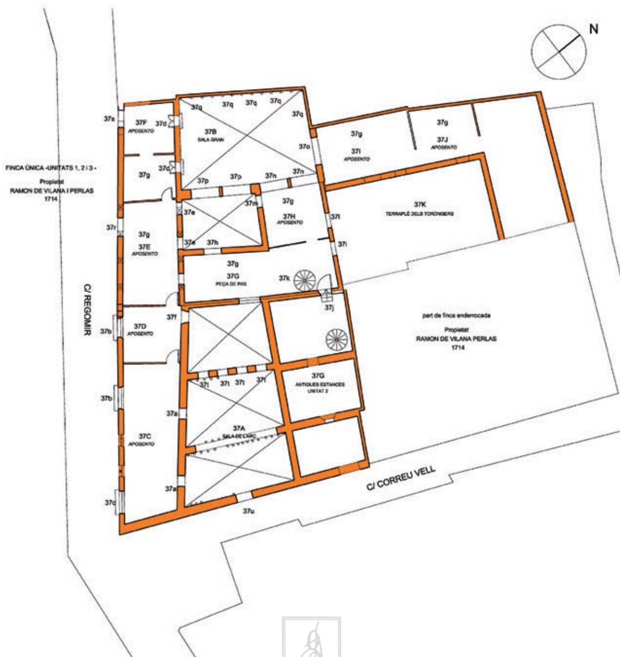
61. Regomir, núm. 11-19. Unitats 2 i 3. Restitució arquitectònica l'any 1714. P. 2a.
