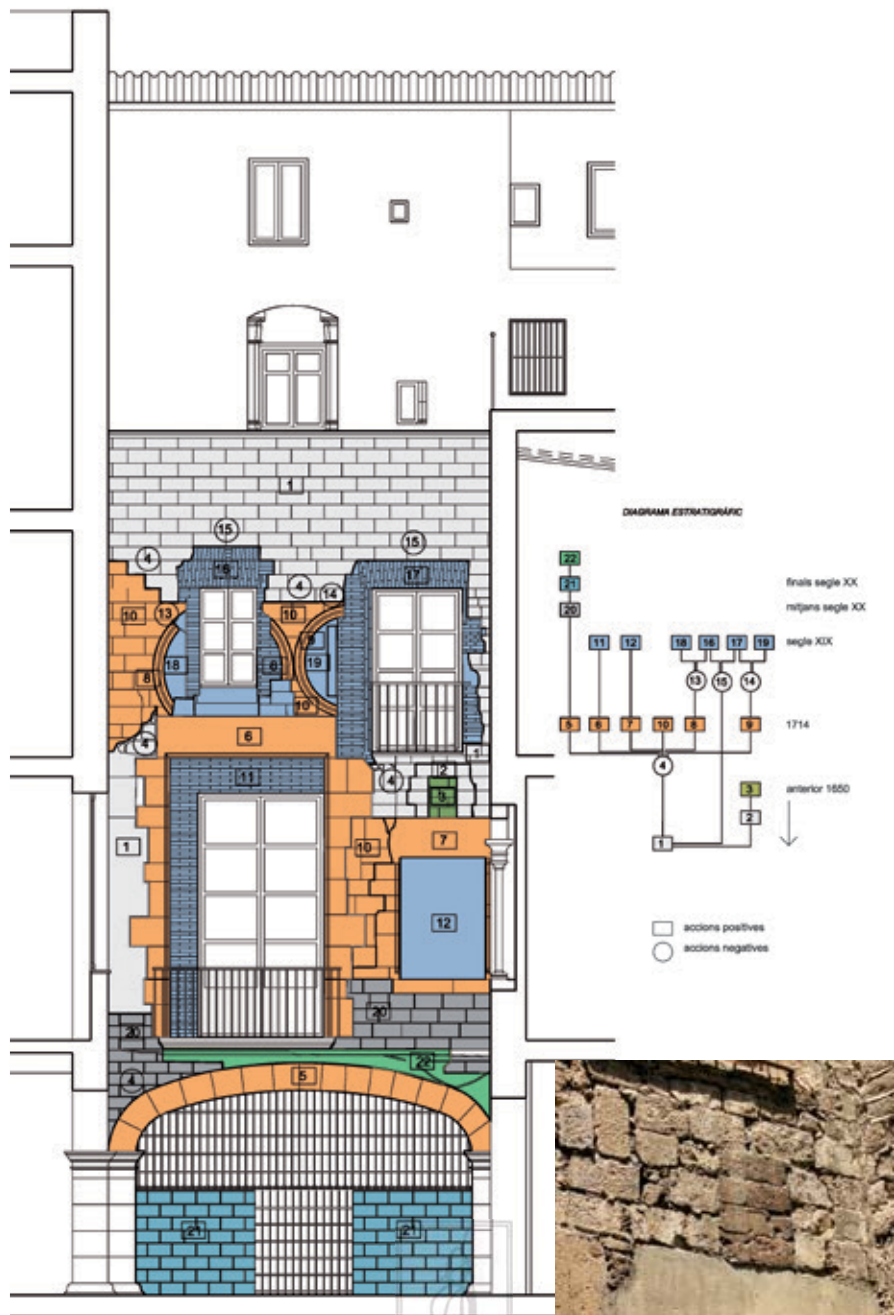
44. Estudi estratigràfic. Accions constructives i diagrama estratigràfic. Cronologia de la construcció. Finestra existent a la planta primera associada a la UE1.
