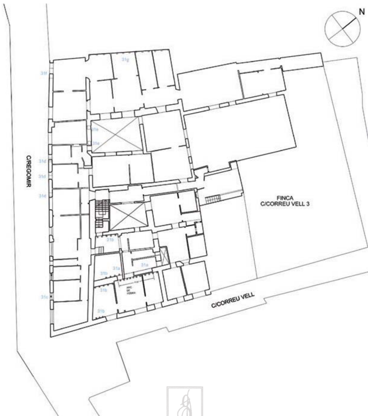
56. Regomir, núm. 11-19. Unitat 2 i 3. Identificació segle XVII sobre l'estat actual. P. 2a.
