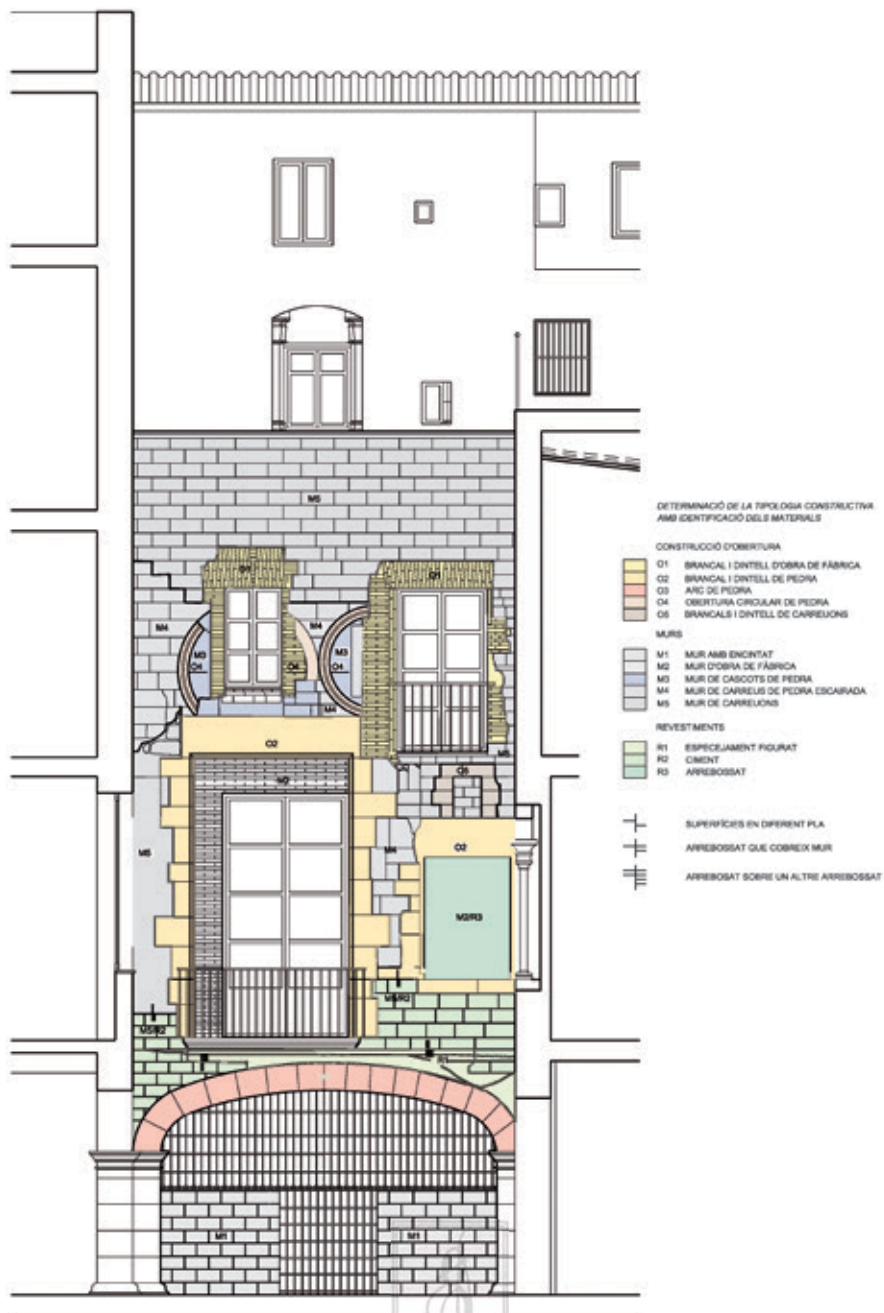
42. Estudi estratigràfic. Determinació de la tipologia constructiva amb identificació dels materials.
