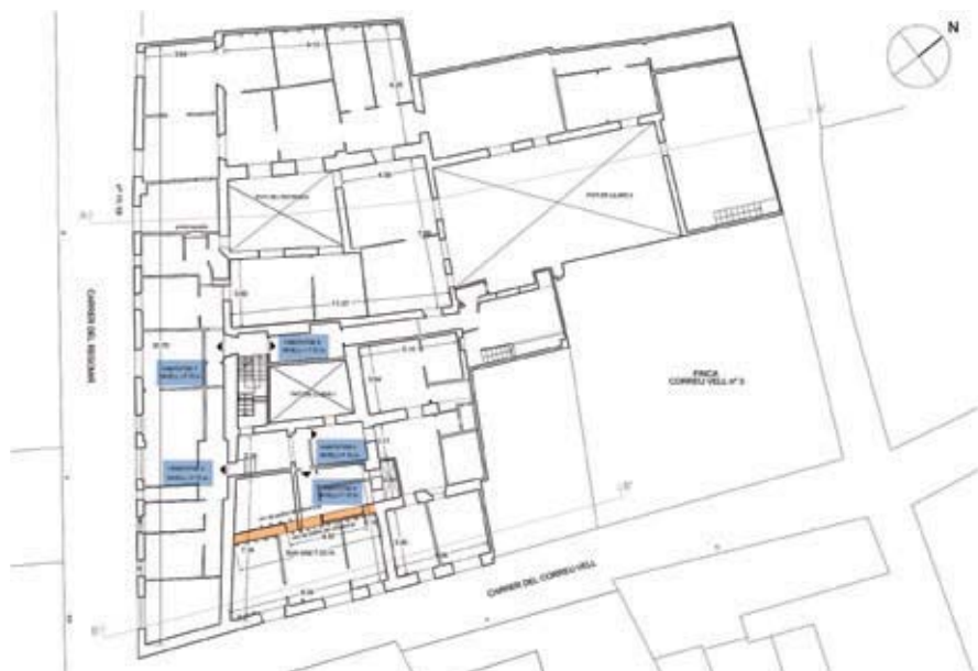
32. Aixecament estat actual. C/ del Regomir, núm. 11-19. Nivell planta segona.
