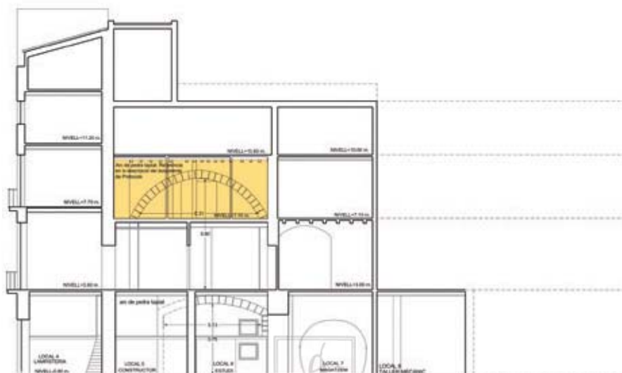
Figura 39. Aixecament estat actual. C/ del Regomir, núm. 11-19. Secció BB'. Vegeu la línia de secció a la figura 30. En aquesta secció s'indica la localització de l'arc corresponent a la gran sala de l'Arc.
