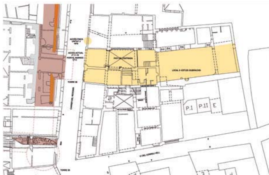
47. Localització d'antic vial anterior al segle xvii. Finca c/ del Regomir; núm. 11-19. Planta baixa.
