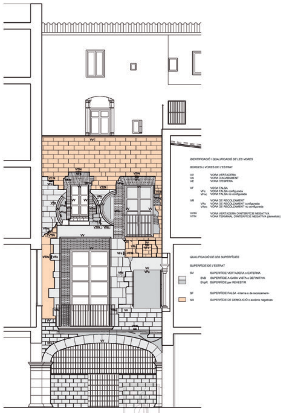
41. Estudi estratigràfic. Identificació i qualificació de vores i superfícies.
