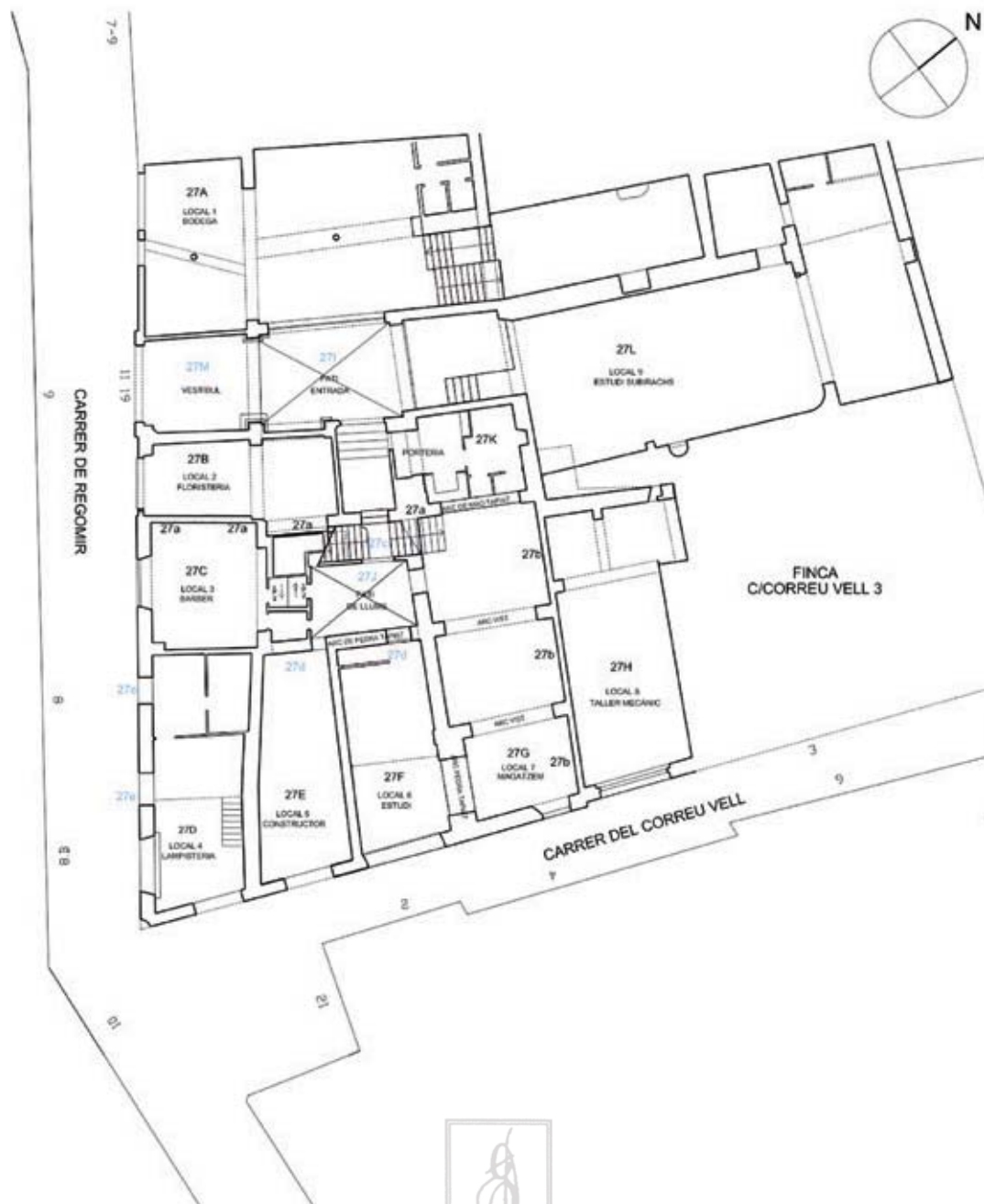
52. Regomir; núm. 11-19. Unitat 2 i 3. Identificació segle XVII sobre l'estat actual. P. B.
