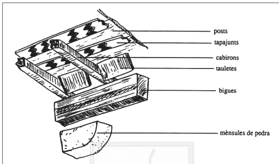
Descripció dels elements de l'embigat de fusta de la planta superior de les naus de l'Hospital de la Santa Creu, elaborat per ARCOR. 1992.
