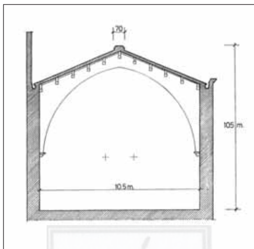
Detalls de la coberta de la planta superior de les naus de Hospital de la Santa Creu.
