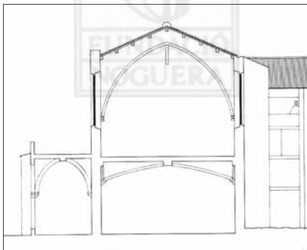
Detalls de les cobertes de les plantes inferior i superior de les naus de l'Hospital de la Santa Creu. Secció transversal. Escala 1:100. 1995.
