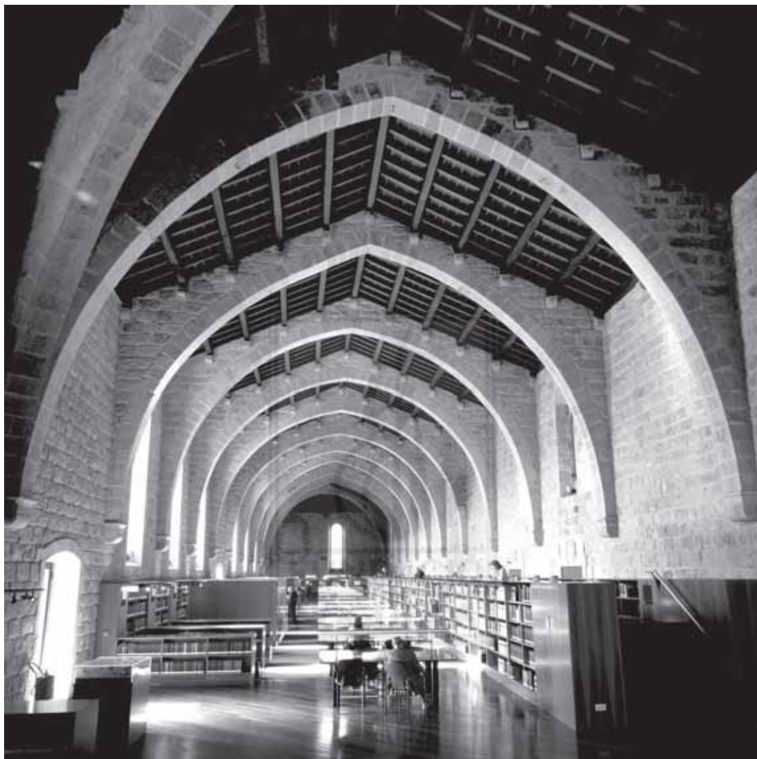
Embigat de fusta de la planta superior de l'Hospital de la Santa Creu. 2005.
