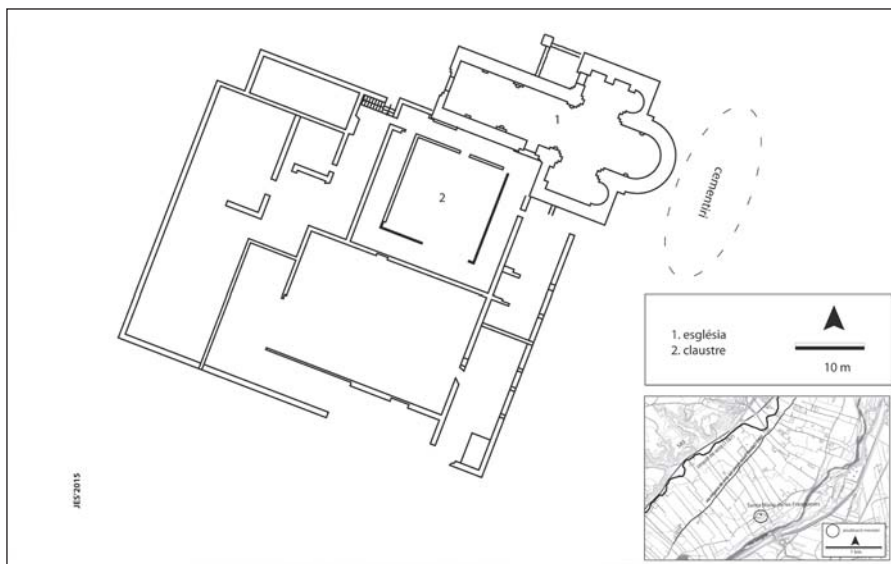
Imatge 4. Planta de les restes conservades de Santa Maria de les Franqueses. 35
