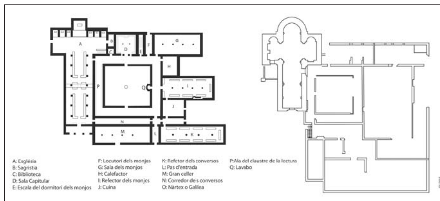
Imatge 5. Planta tipus i planta del monestir de Santa Maria de les Franqueses.
