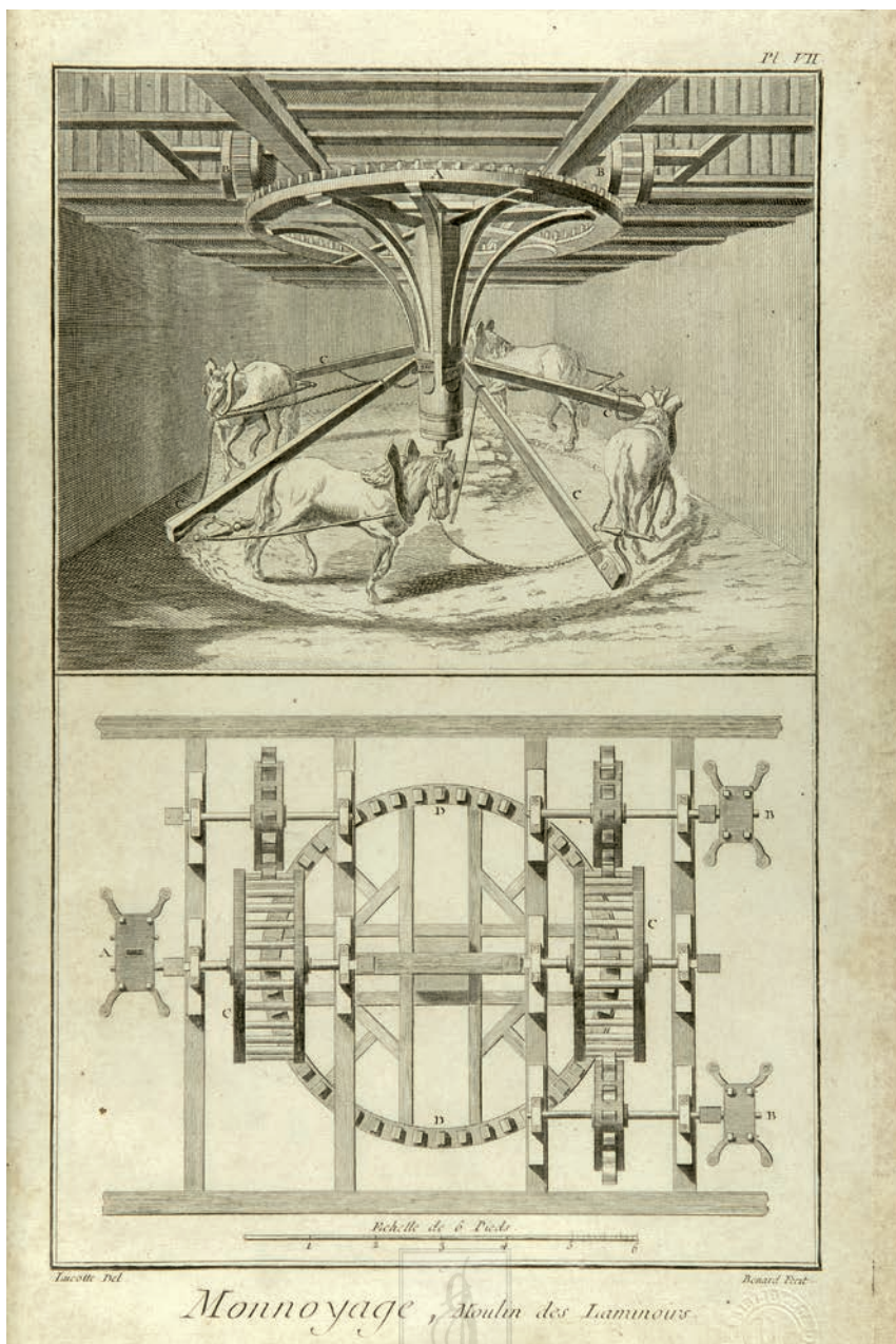
15. Molí mogut a sang destinat a laminar el metall que s'ha d'encunyar. Gravat que il·lustra l' Encyclopédie francesa, 1765. © Biblioteca de Catalunya, Barcelona.
