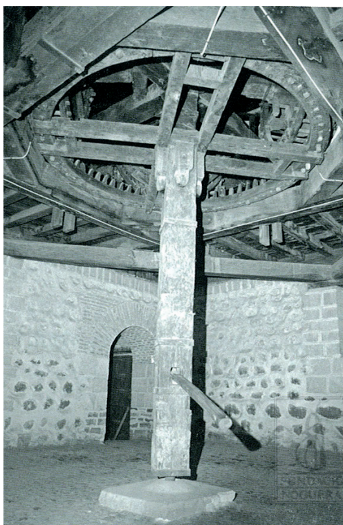
16. Part superior i inferior del molí de laminació mogut a sang de la seca de Potosí, segle XVIII. © Museo Casa de la Moneda, Potosí.
